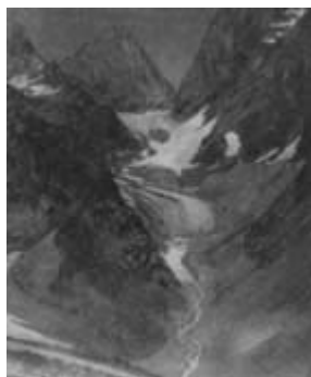
Котел Аксаутского ледника в глубине Марухкая
